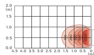
EU-7RS/EU-7GS/EU-7RS-F
