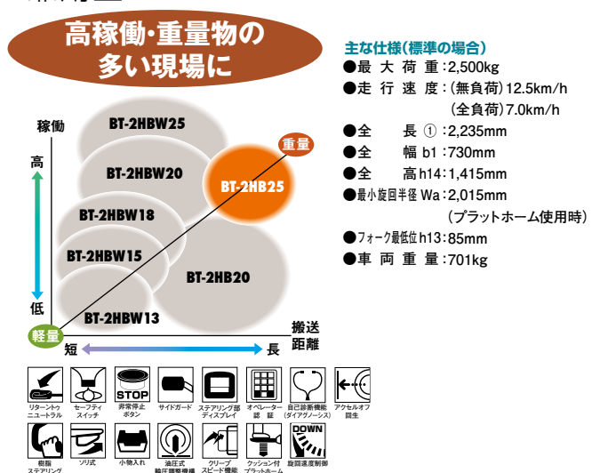
乗車・歩行 兼用型2.5t BT-2HB25
