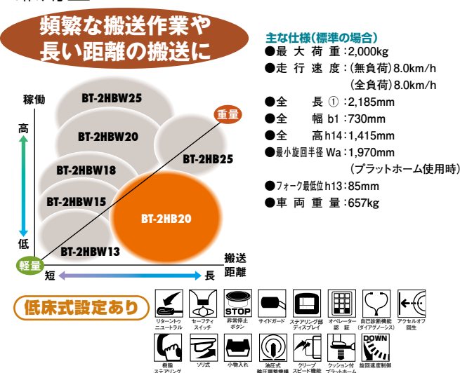
乗車・歩行 兼用型2.0t BT-2HB20
