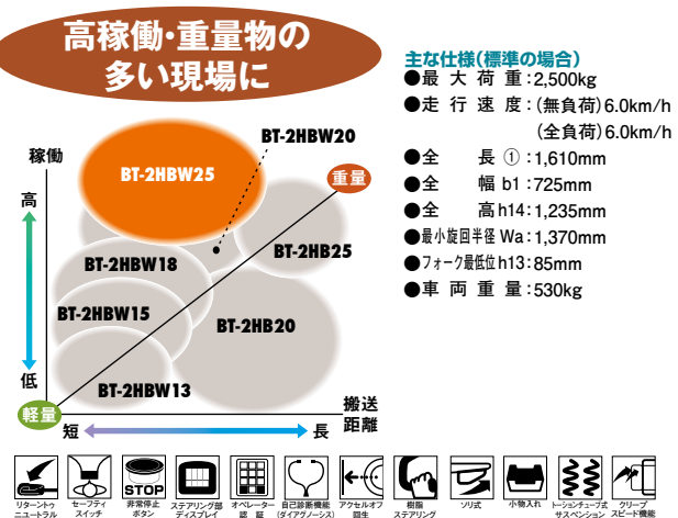
步行型2.5t BT-2HBW25
